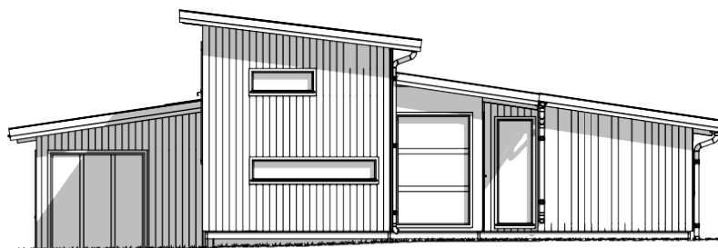
FasadA2 1:50
